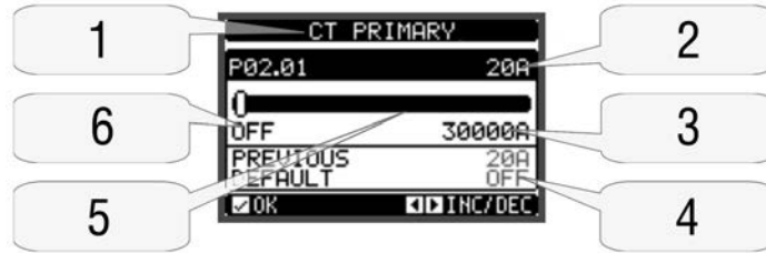
Настройка: страница изменения значений параметров
