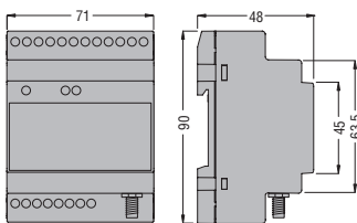
MODEM GSM PER COMANDO A DISTANZA E MONITORAGGIO VIA SMS EXCGSM01
