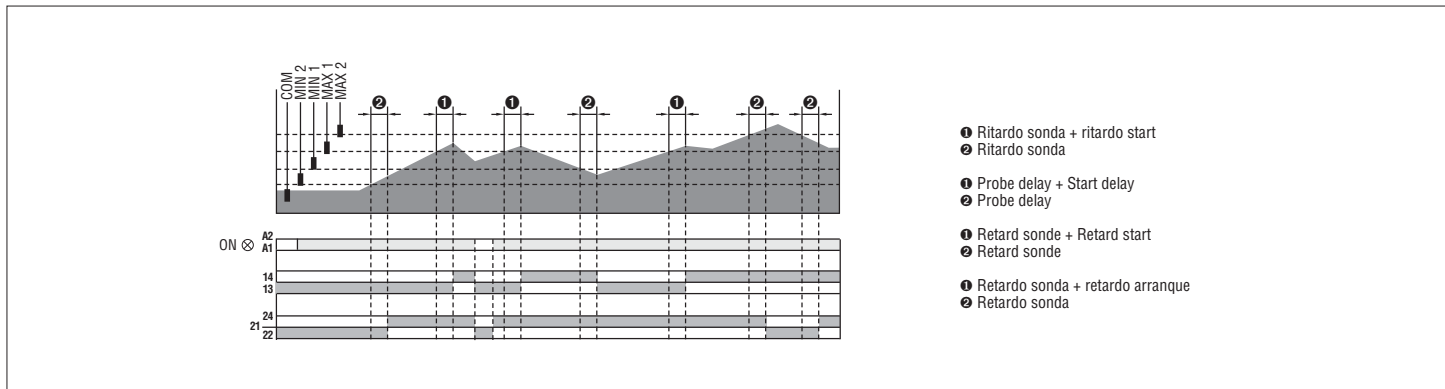
DIAGRAMMA DI FUNZIONAMENTO (Modo A)
