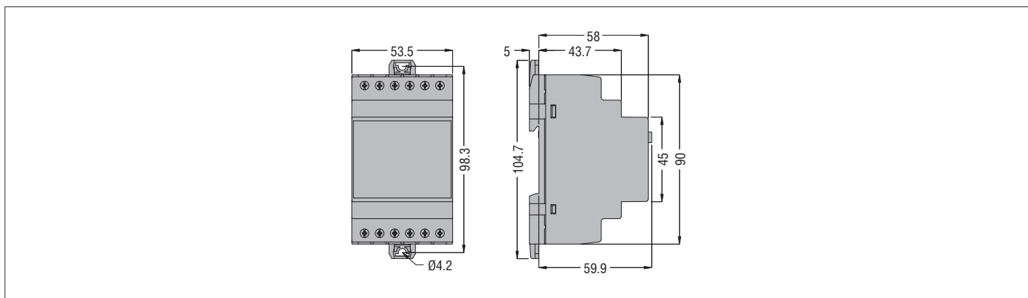
DIMENSIONI MECCANICHE [mm]
